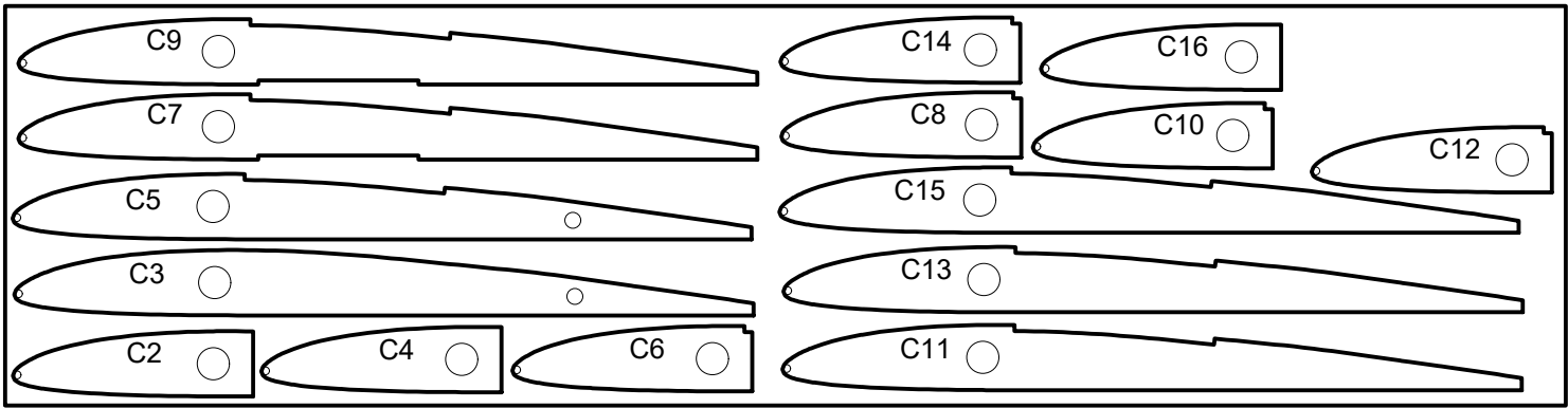
REBRA CENTROPLANA (balza 2 mm)
