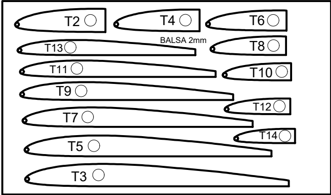
REBRA TERMINEZONA (balza 2 mm)
