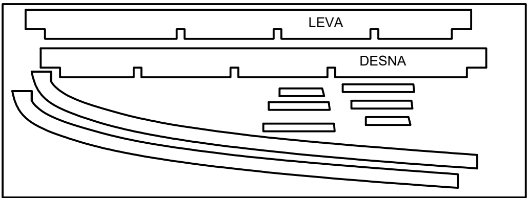
VIŠINSKI STABILIZATOR (balza 3 mm)
