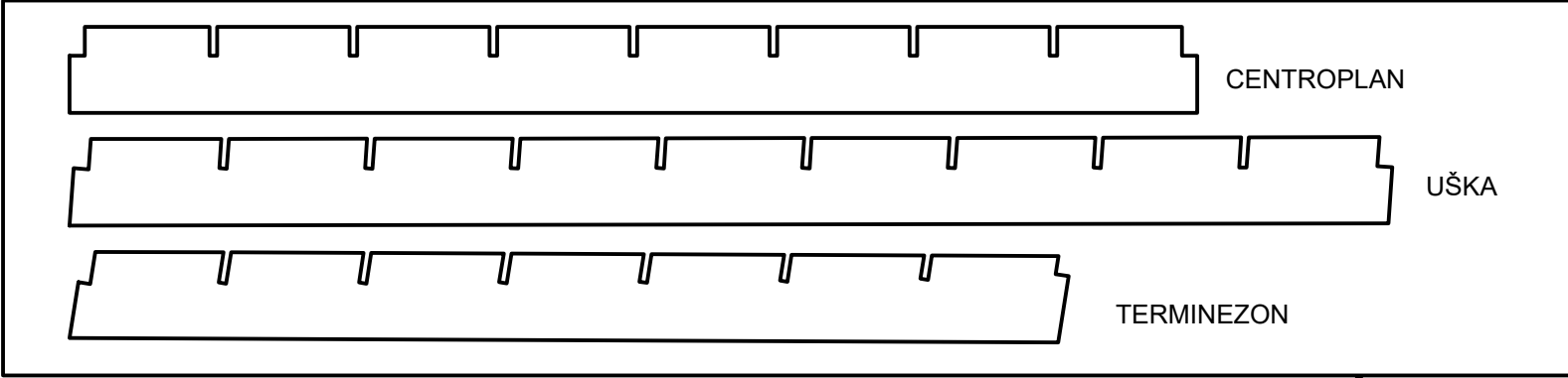
ZADNJI ROBOVI KRIL (balza 3 mm)
