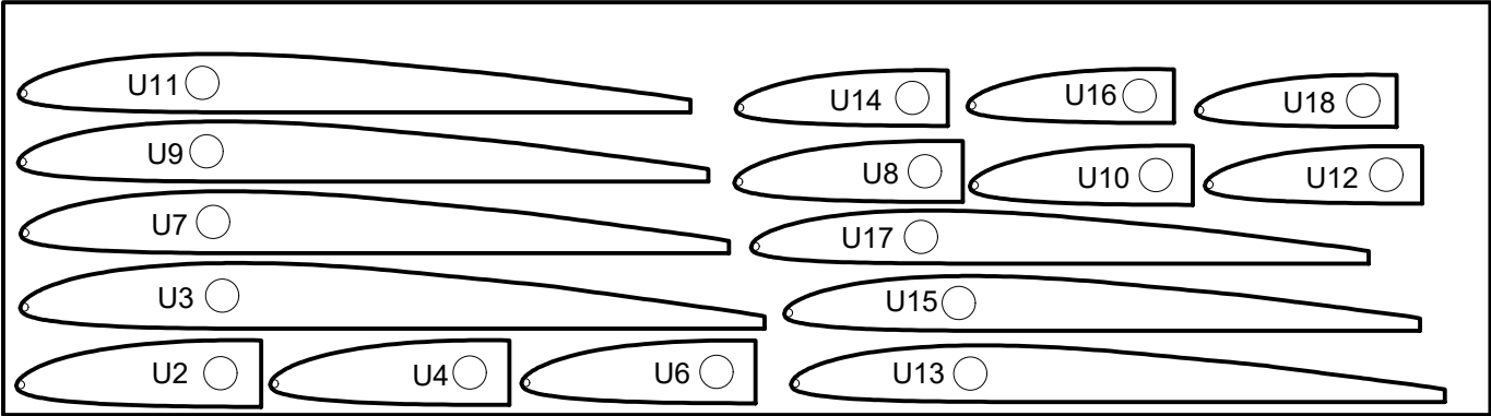
REBRA UŠK (balza 2 mm)
