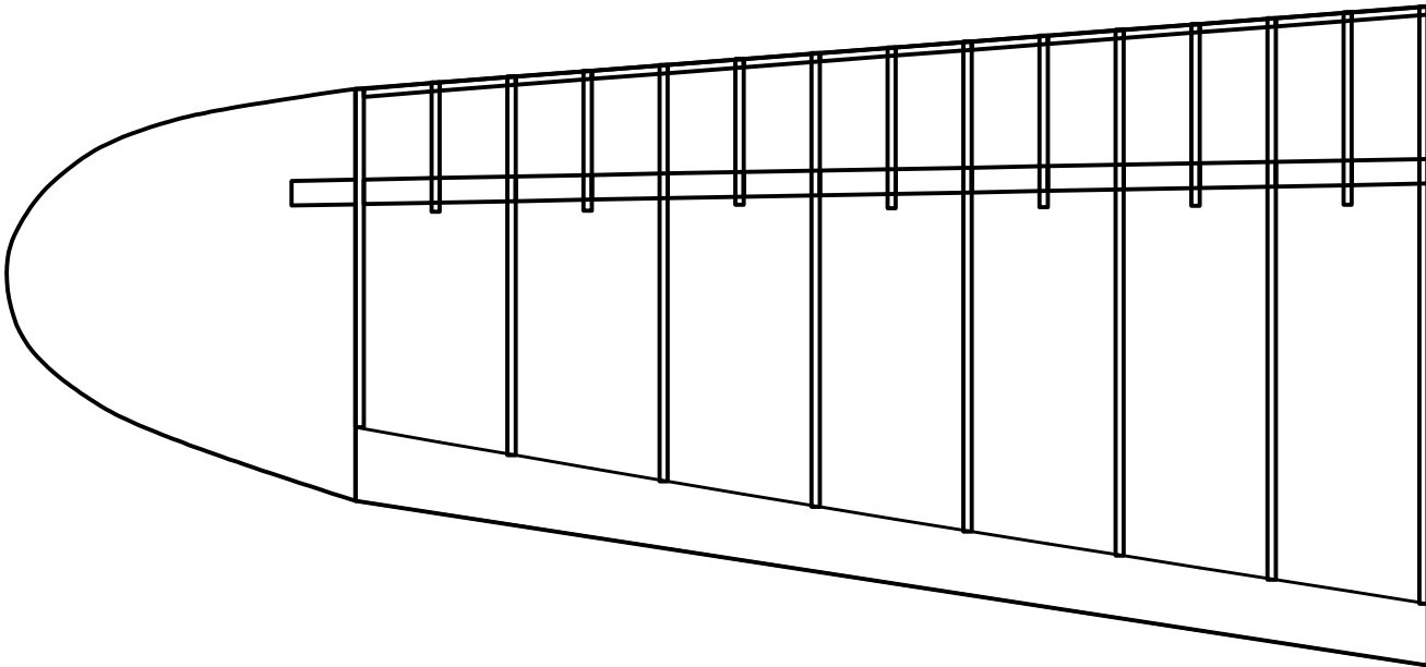
ŠABLONA ZA LEVI TERMINEZON
